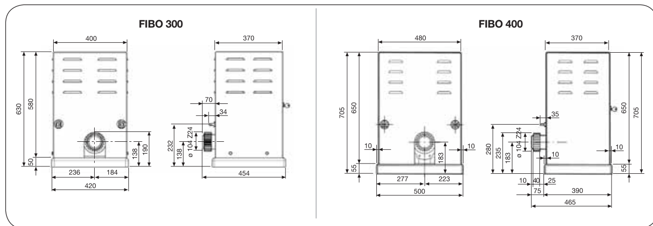
Binnenaanzicht FIBO 300 en FIBO 400 met geïnstalleerd krachtschakelpaneel
